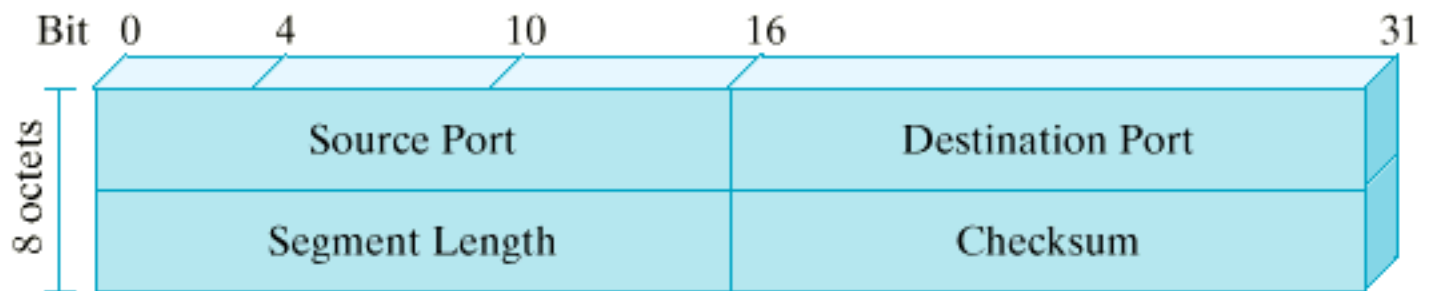
(b) UDP Header
